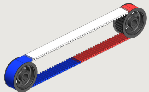
Exemple d'assemblage d'une longueur de 3360 mm avec 3 sections de 1120 mm
